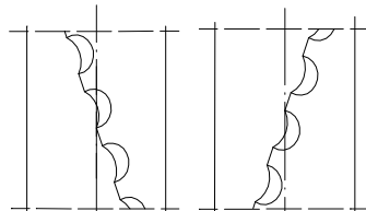
Linksspiralig left twisted
